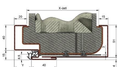
Obložková renovační zárubeň OZ
