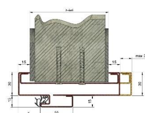
Dvoudílná variabilní zárubeň DSv
