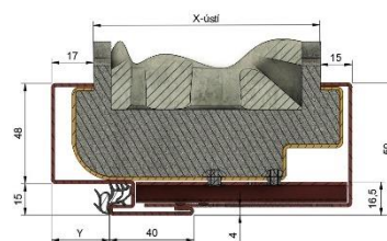
Obložková renovační zárubeň OZO
