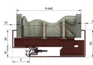
Dvoudílná zárubeň DZD
