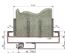
Dvoudílná zárubeň DS
