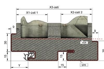
Zárubeň UDF – DZD
