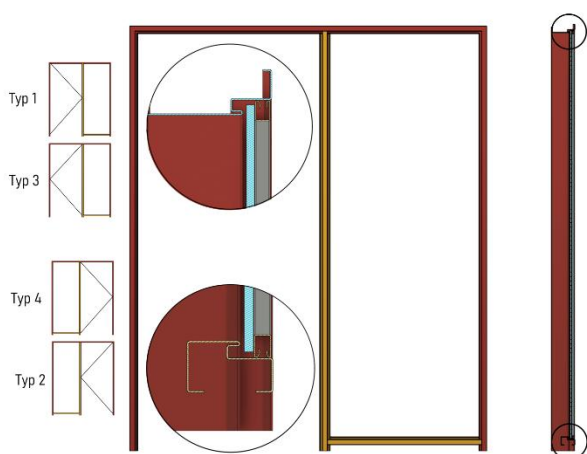
Zárubeň LZ s postranním světlíkem pro jednostranné zasklení
