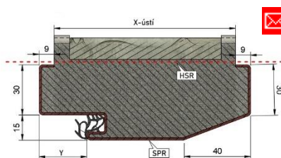
Nemocniční zárubeň N
