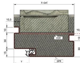
Světlíková zárubeň s dvojítm f. SDF
