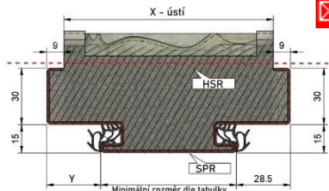
Dvou dveřní zárubeň DDZ
