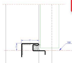
Profil č. 60 - pro rozdílné výšky podlah
