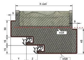
Rohová renovační zárubeň RR
