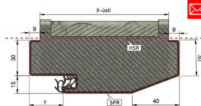
Nemocniční zárubeň N
