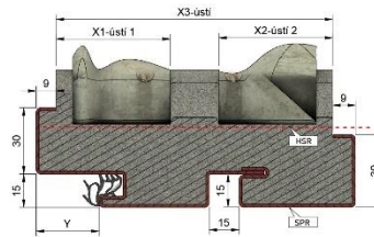
Zárubeň UDF - DZD
