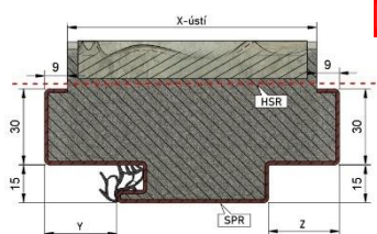
Dvou dveřní zárubeň DDZ
