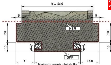
Dvou dveřní zárubeň DDZ
