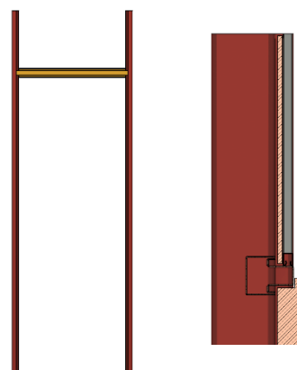
H - zárubeň s nadsvětlíkem
