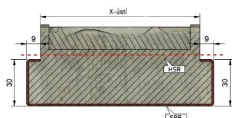
Rohová zárubeň RP
