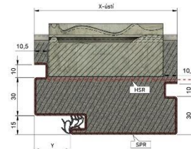
Světlíková zárubeň s dvojitém f. SDF
