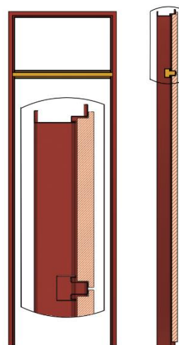
Zárubeň pro naddveňní panel s dělicím profilem
