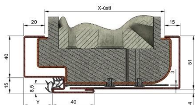
Zárubeň USD - DZD
