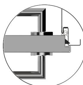
Zárubeň a dveře "s polodrážkou" (falcové)
