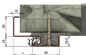
Zárubeň s optickou polodrážkou OP
