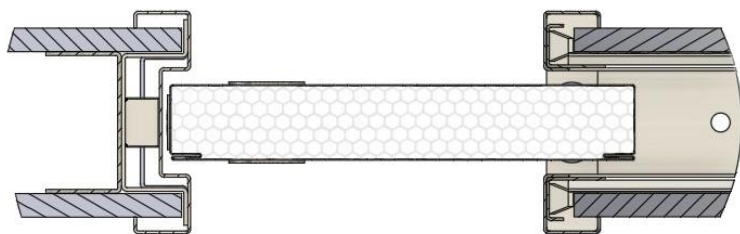
Posuvné zárubně ve zdi jdoucí
