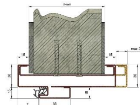
Obložková renovační zárubeň OZO
