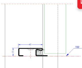
Profil č. 55 - pro dodatečnou montáž
