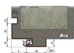
Rohová zárubeň se stín. dr. RSD
