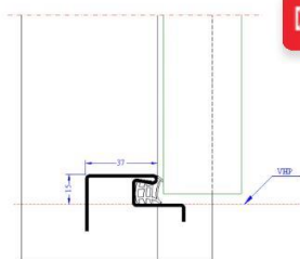
Profil č. 55 - pro dodatečnou montáž
