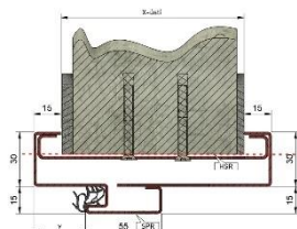
Obložková renovační zárubeň OZ
