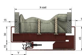
Dvoudílná zárubeň DZD
