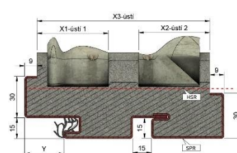
Dilatační zárubeň DLZ
