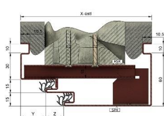
Zárubeň USD - UDF - DZD
