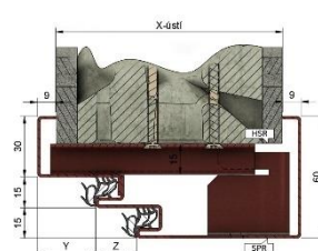
Zárubeň UDF - DZD
