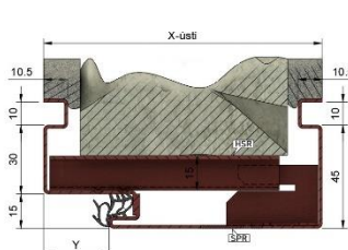
Zárubeň USD - UDF - DZD
